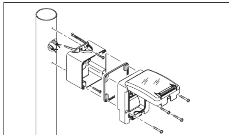
Единична кутия за монтаж странично стълб с до Ø 70mm (включен е и адаптор за Ø 50mm)
