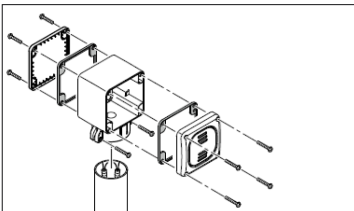
Единична (и двойна) кутия за монтаж върху тръба с Ø 60mm (включен е и адаптор за Ø 50mm)
