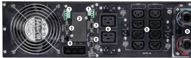
Eaton 9PX 6 kVA 1:1
