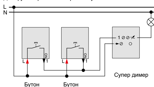
Димируема кръстат верига с бутон
