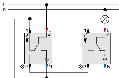
Девиаторен ключ с индикаторна лампа Девиаторен ключ с индикаторна лампа
