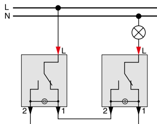
Девииаторен ключ с глим лампа Девииаторен ключ с глим лампа
