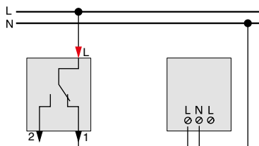
Девииаторен ключ
