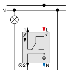
Девииаторен ключ с индикаторна лампа
