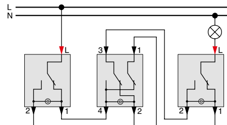
Девииаторен ключ с глим лампа Кръстат ключ с глим лампа Девииаторен ключ с глим лампа
