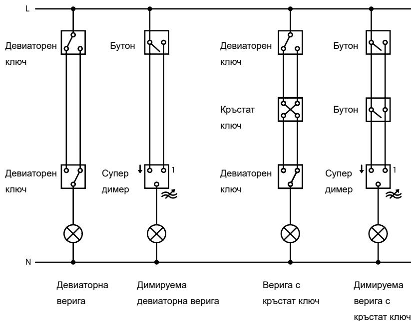
Димиране на осветителни тела
