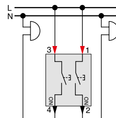
Двоен бутон нормално отворен
