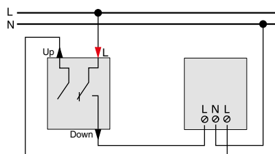
Ключ за управление на ролетни щори
