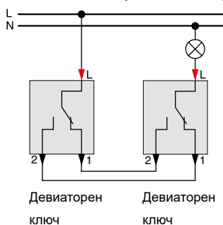
Схема на съществуваща девиаторна верига
