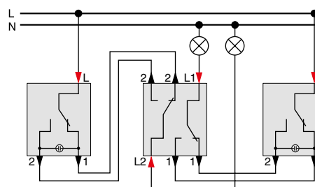
Девииаторен ключ с глим лампа Двоен девиаторен ключ Девииаторен ключ с глим лампа
