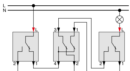
Схема на съществуваща верига с кръстат ключ
