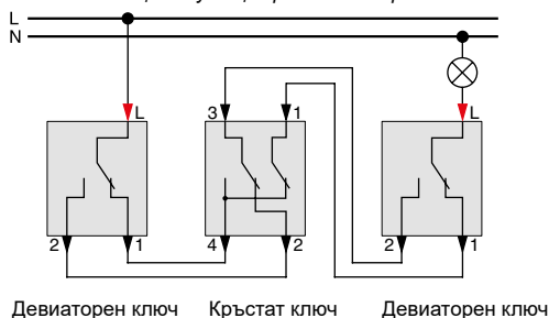
Схема на съществуваща кръстат верига
