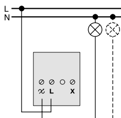
Схема с димиране на осветителни тела
