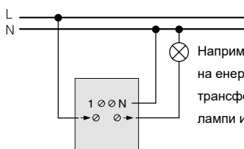
Схема с универсален релеен механизъм
