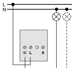
Ротативен димер
