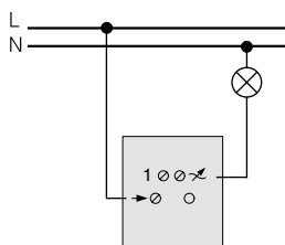
Схема с електронен ключ
