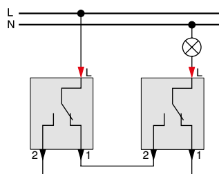
Схема на съществуваща верига с девиаторни ключове
