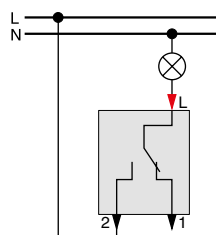
Схема със съществуваща верига с еднополюсен ключ
