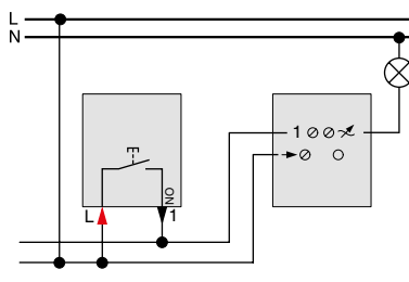
Схема с димируема девиаторна верига с бутон
