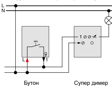
Димируема девиаторна верига с бутон
