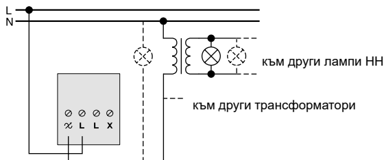
Ротативен димер
