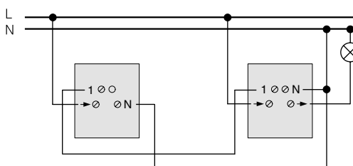
Схема с релееен ключ и механизъм TELE разширение
