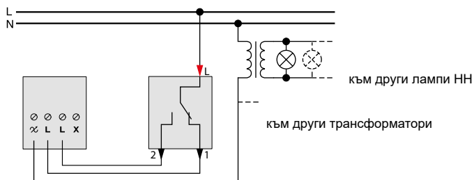
Ротативен димер
