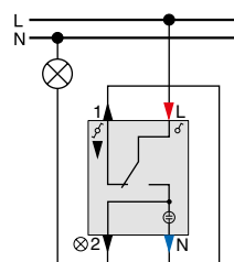
Девииаторен ключ с индикаторна лампа
