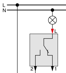
Еднополюсен/девиаторен ключ
