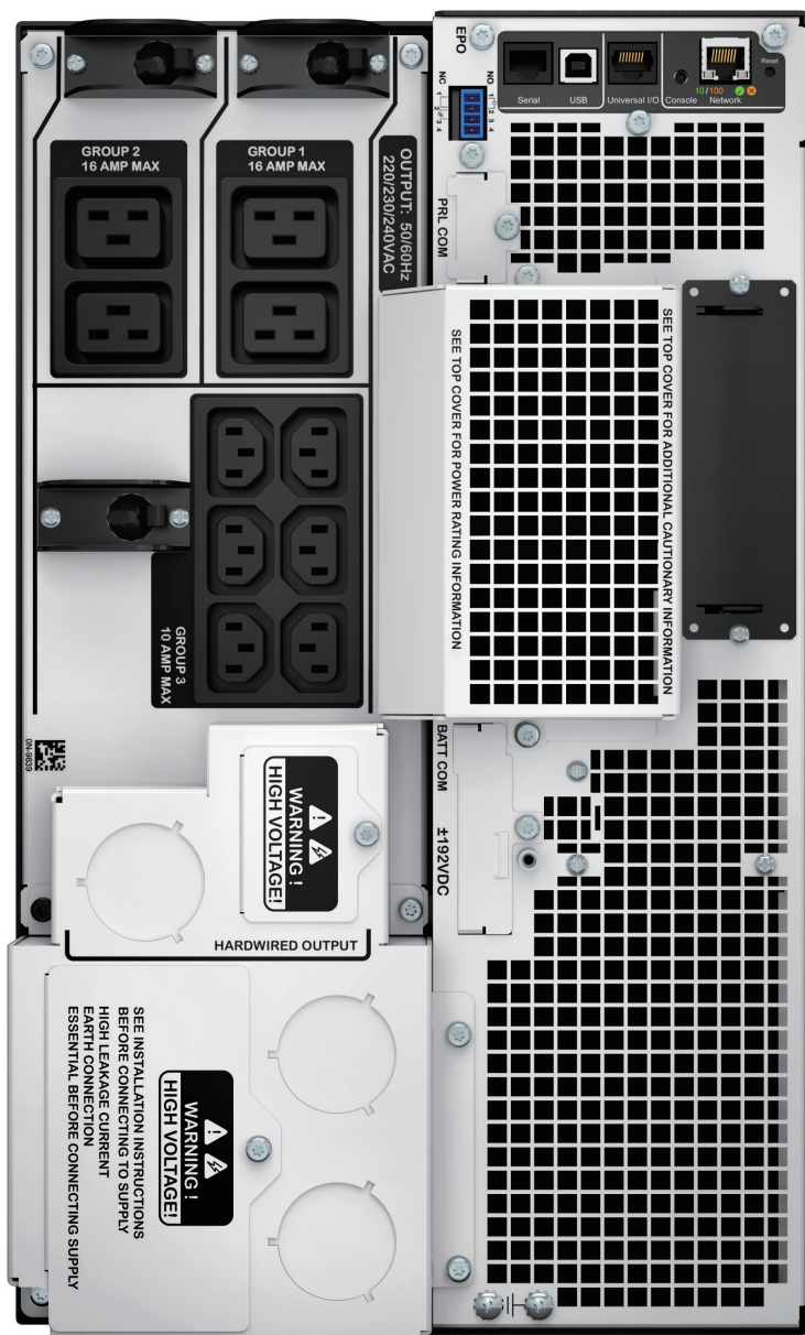
SRT10KXLT shown
